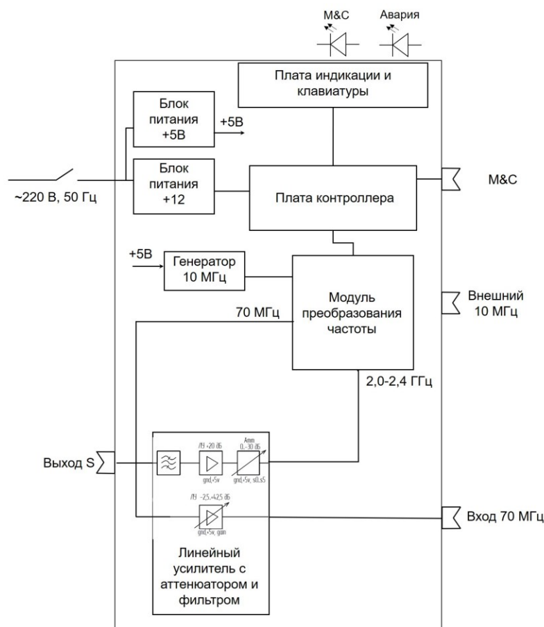
Рисунок 2 – Структурно-функциональная схема ПЧ «вниз»
